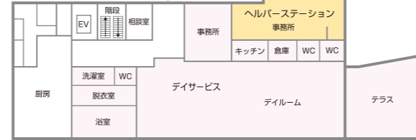
1階平面図
